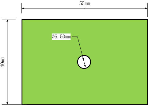
图 2.4 电梯轿厢端控制器读卡头尺寸图
