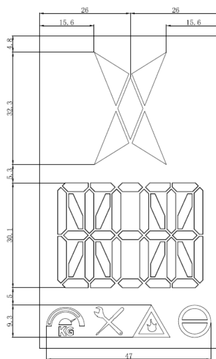
屏显尺寸图
