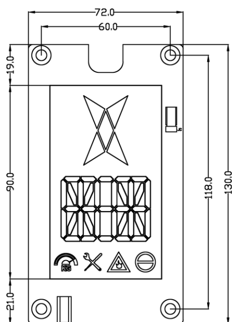
正面尺寸图
