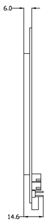
侧面尺寸图
