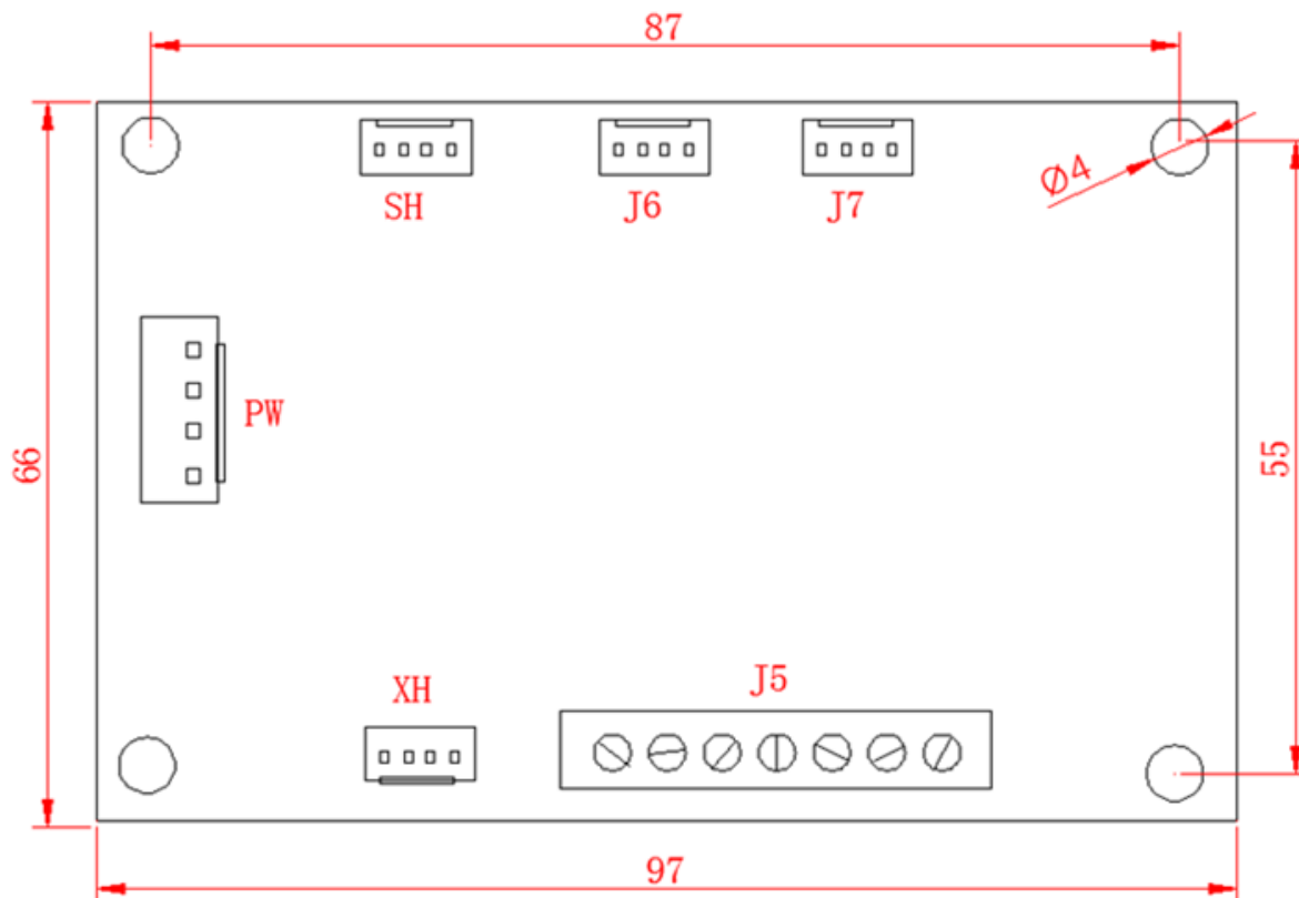
正面尺寸图
