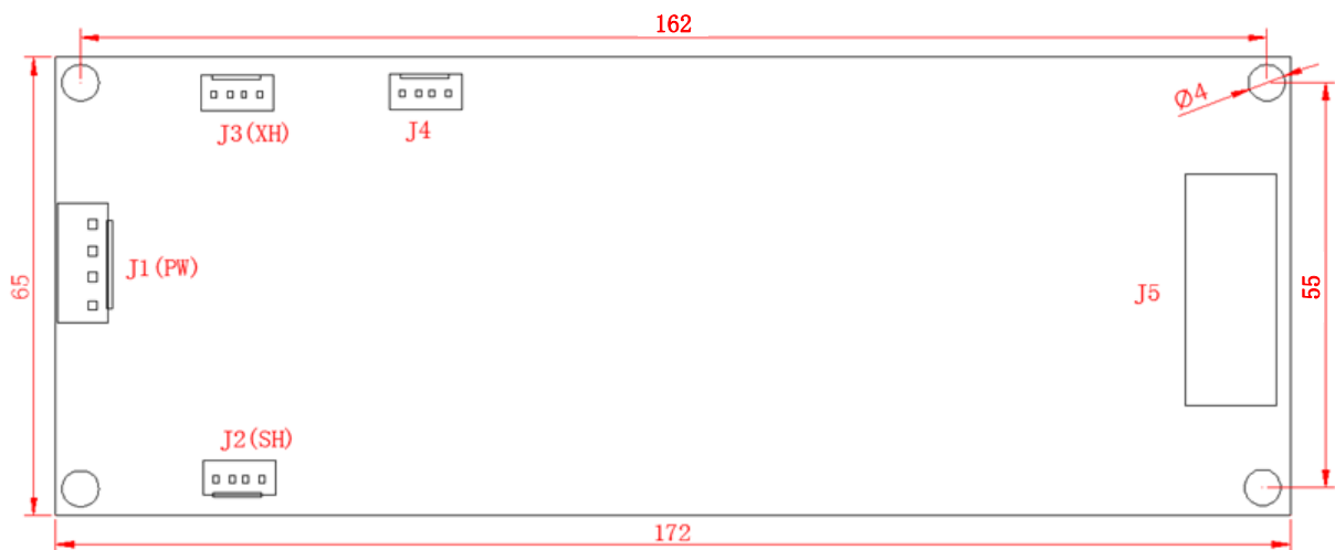
图 2.4 BL2000-HXK-V9 尺寸图 (单位 mm)
