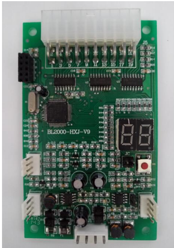
图 2.1 BL2000-HXJ-V9 实物图
