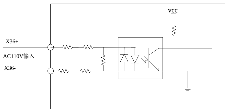
图 3.10 AC110V 输入接口原理及接线示意图
