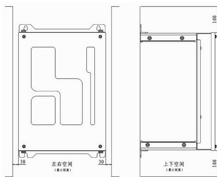
图 2.11 安装方向和安装空间示意图
