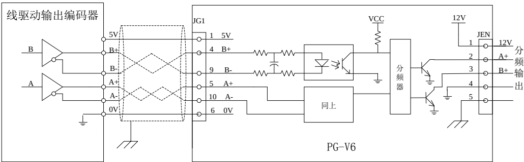
图 3.13 PG_V6 卡与 5V 线驱动输出编码器连接示意图(异步电机使用)
