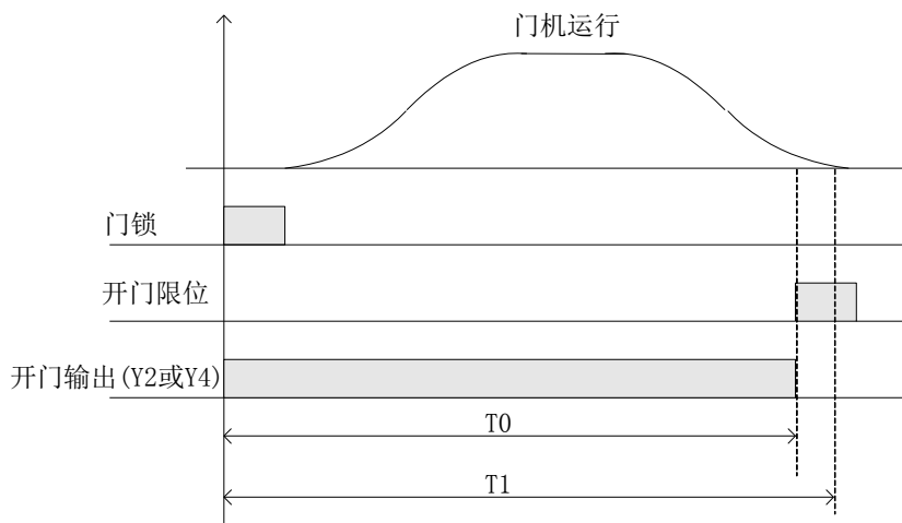
图 6.7 开门时序图
