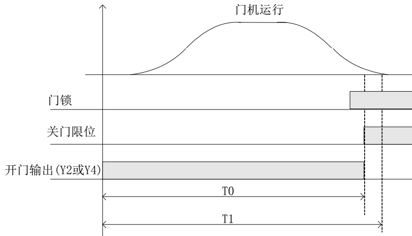
图 6.8 关门时序图
