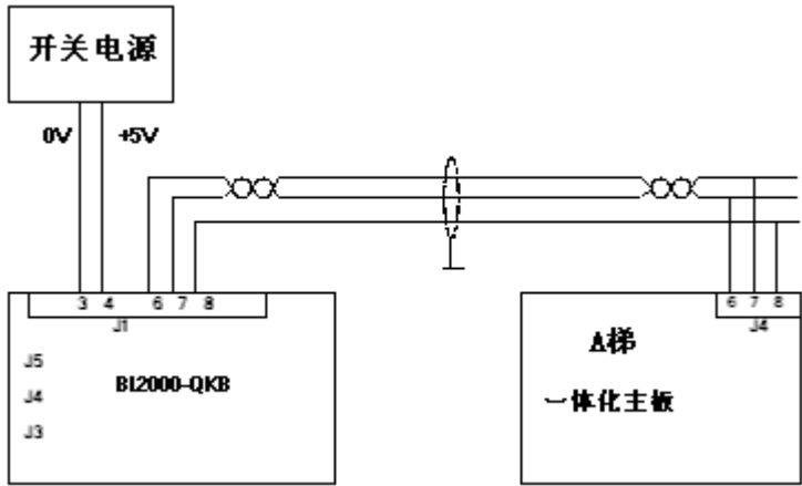
图 11.2 群控电脑板 BL2000-QKB-V1 接口电路图
