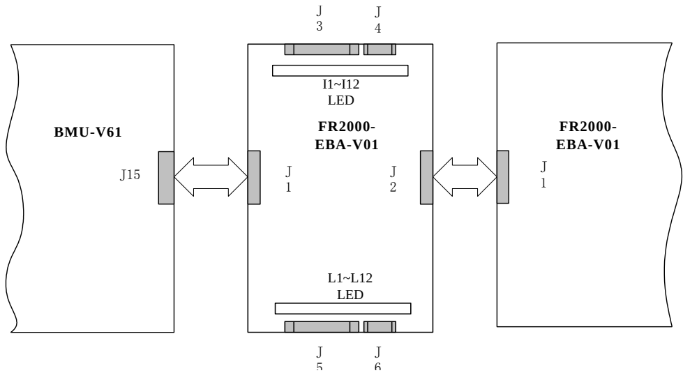
图 11.4 并行扩展板 FR2000-EBA-V01 接口电路图
