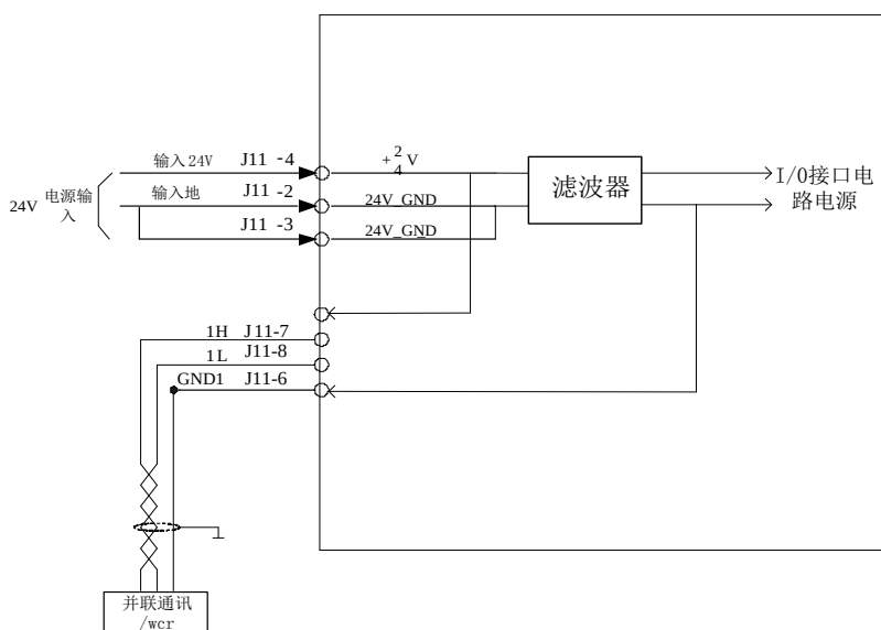
图 3.11 电源接口原理及配线示意图
