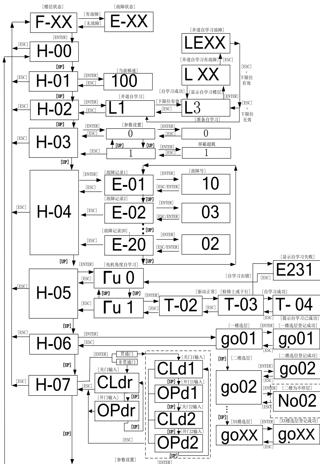
图 F4.1 主控板数码块与按键配合设置流程图
