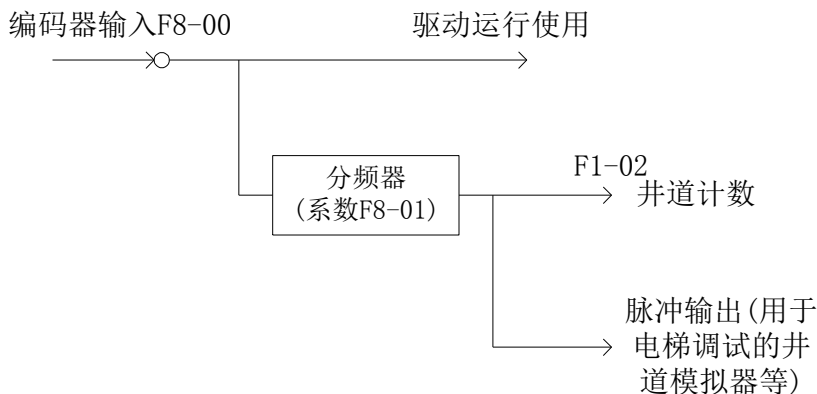
图 6.15 编码器脉冲使用分布图
