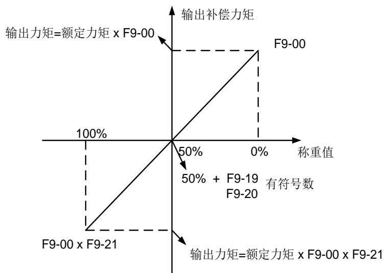
图 1.6.1 称重原理框图
