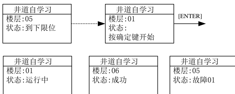
图 1.5.1 井道自学习操作示意图
