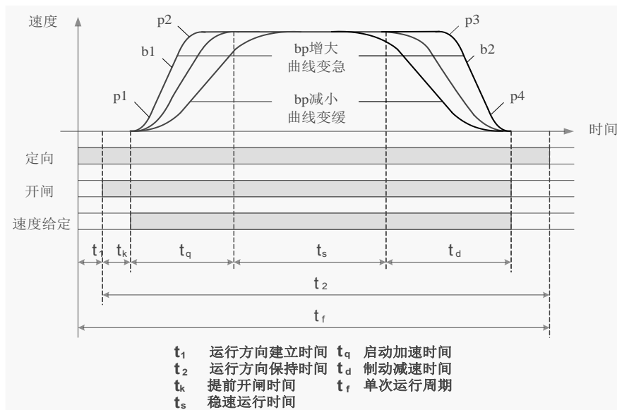
图 1.6.3 运行曲线示意图
