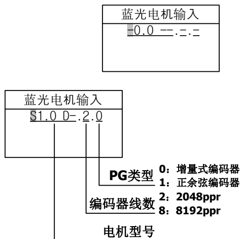
图 6.1.1 蓝光电机输入界面
