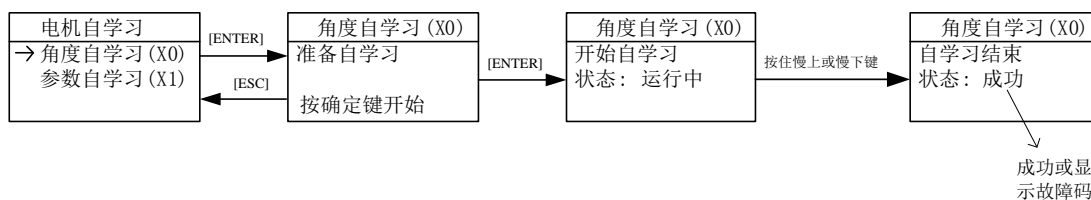
图 6.2.2 负载（带钢丝绳）角度自学习操作示意图
