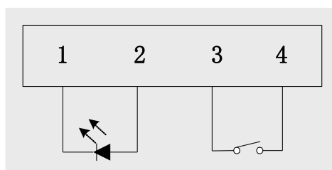
图 5.2 内选按钮接线图
