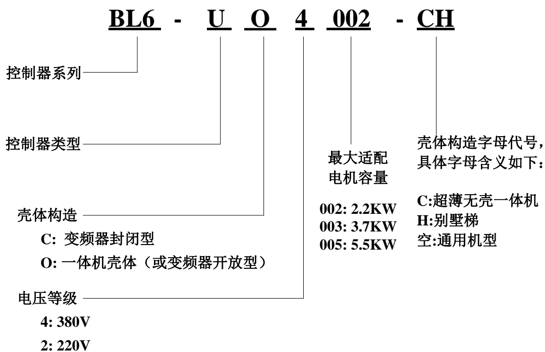
图 1.1 型号说明示意图
