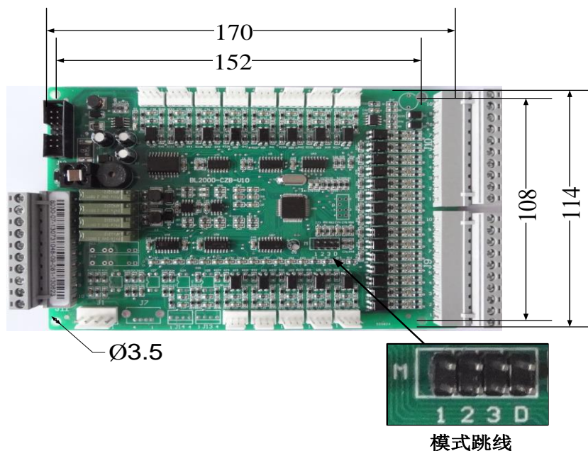
图 5.1 操纵盘板 BL2000-CZB 示意图
