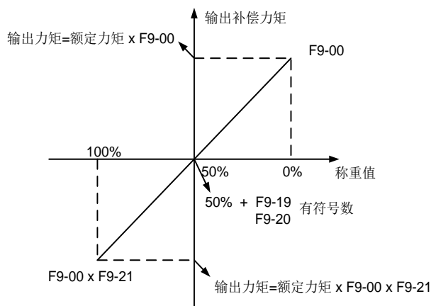
图 6.6.1 称重原理框图
