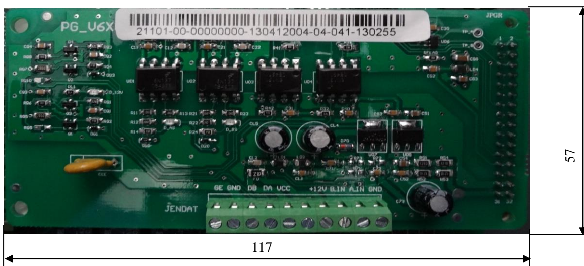
图 4.2 PG_V6X 接口卡外形及平面安装尺寸
