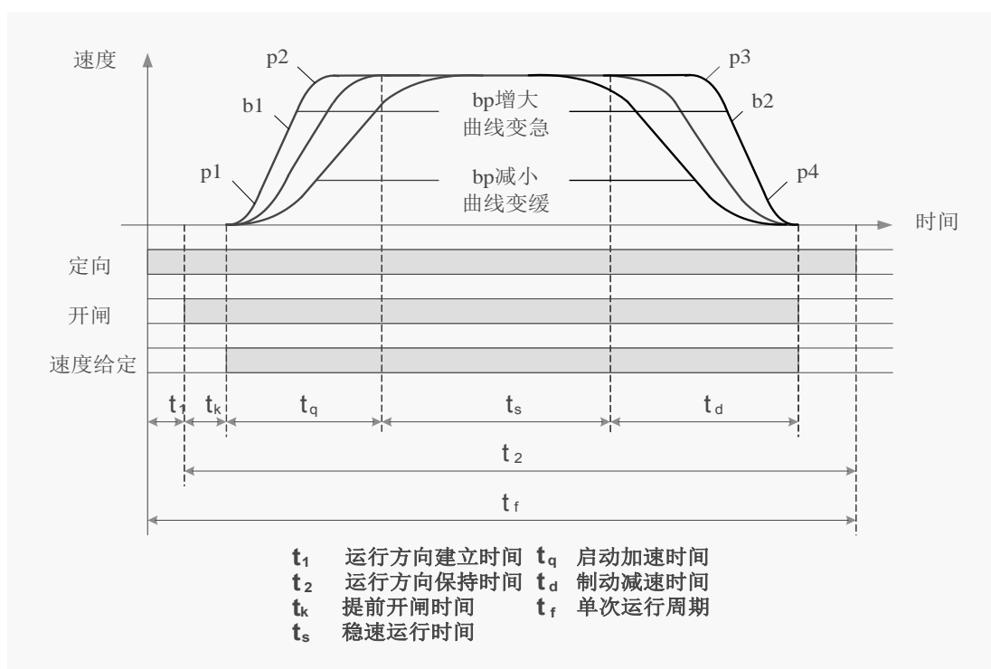
图 6.6.3 运行曲线示意图
