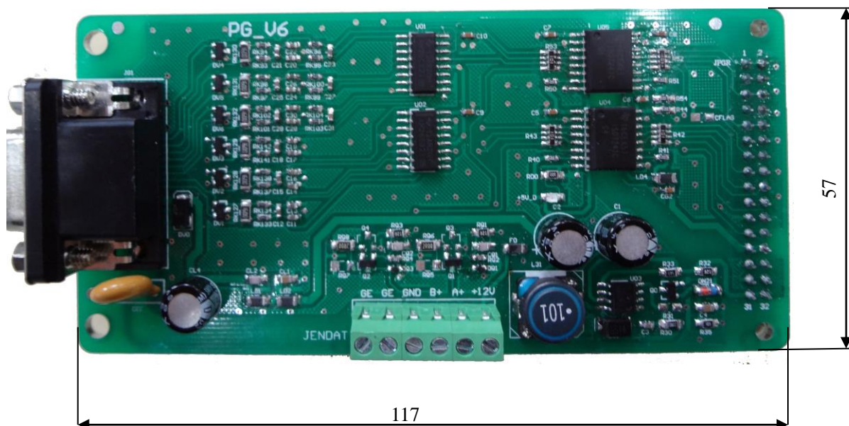
图 4.1 PG_V6 接口卡外形及平面安装尺寸
