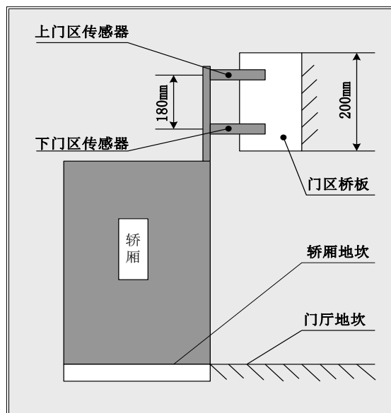
门区开关与门区桥板安装示意图
