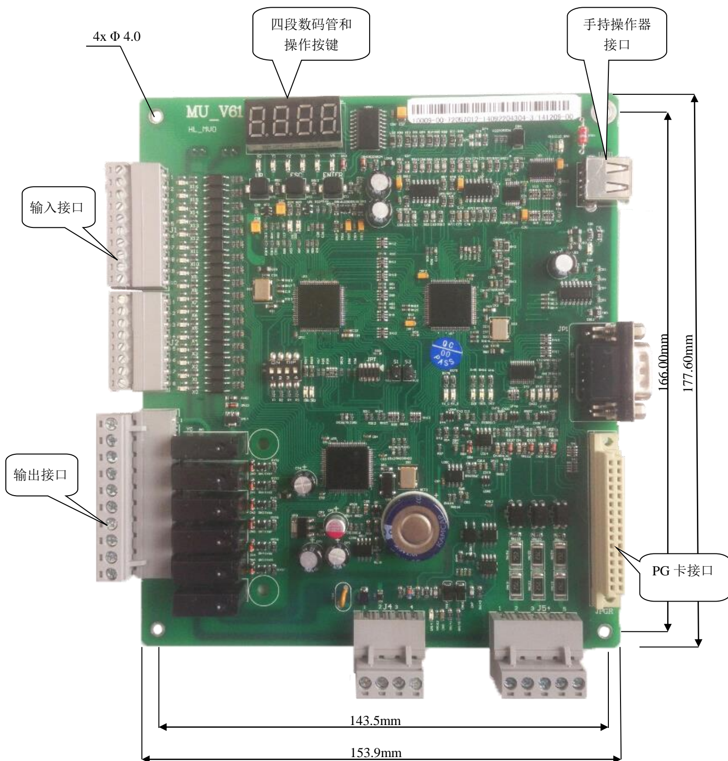
图 3.1 主控板端子位置示意图
