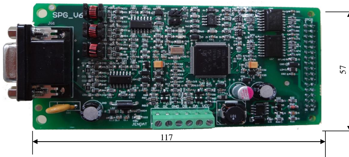
图 4.3 SPG_V6 接口卡外形及平面安装尺寸
