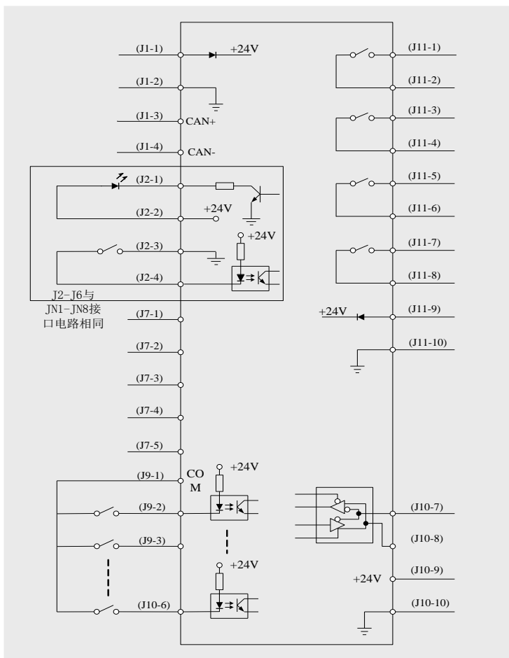
图 5.4 轿厢电脑板 BL2000-CZB 接口电路图
