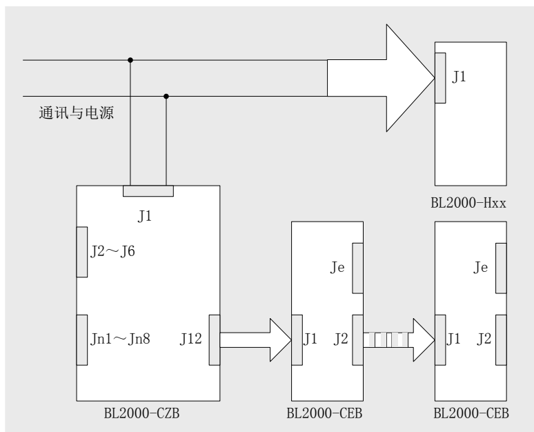
图 5.3 轿厢电脑板与轿厢扩展板连接图
