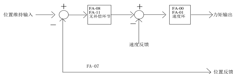
图 6.6.2 无负载补偿起动的原理示意图
