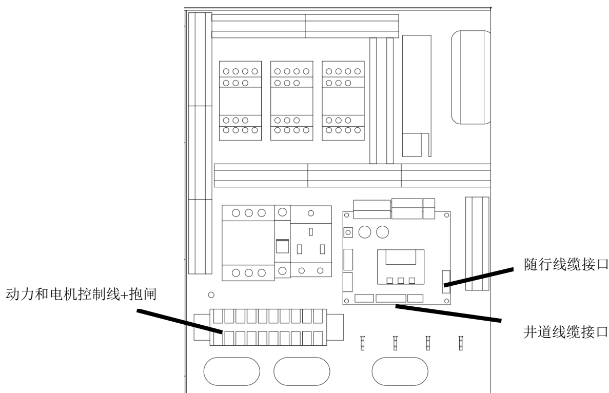
图 3.1 控制柜内部对外接线示意图
