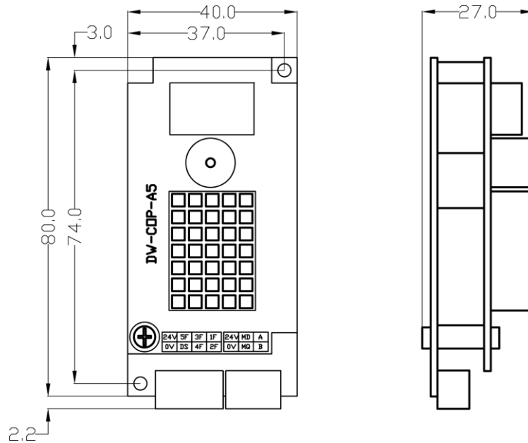
图 6.1 DW-COP-A5 尺寸图
