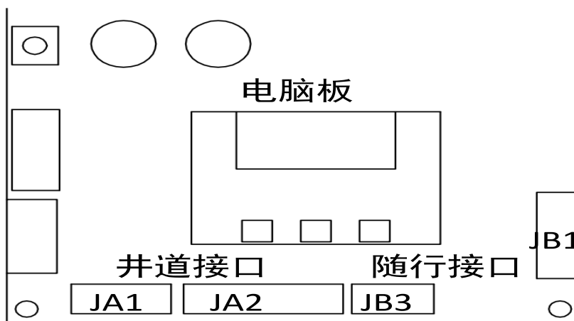
图 3.3 随行和井道端子示意图
