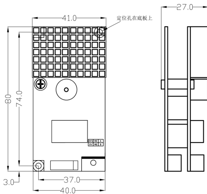
图 6.2 DW-COP-A15 尺寸图
