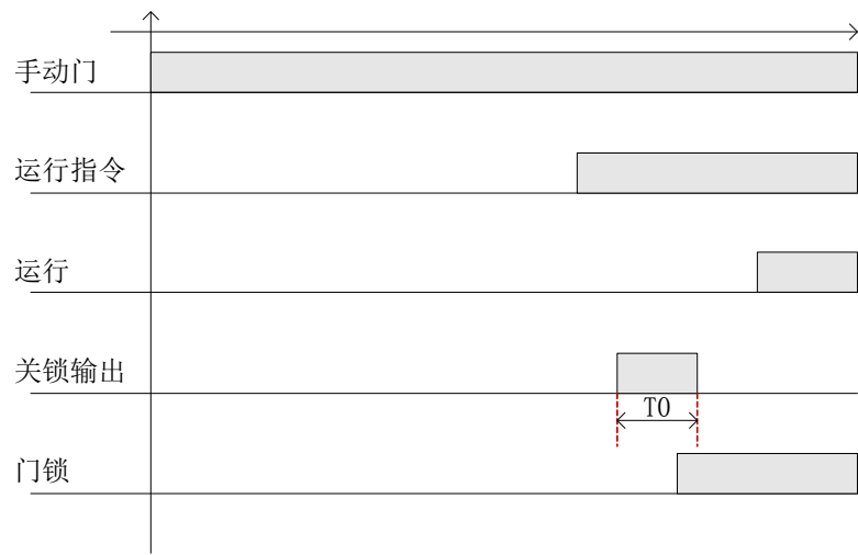
图 6.10 门锁吸合时序图
