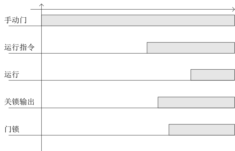
图 6.8 门锁吸合时序图
