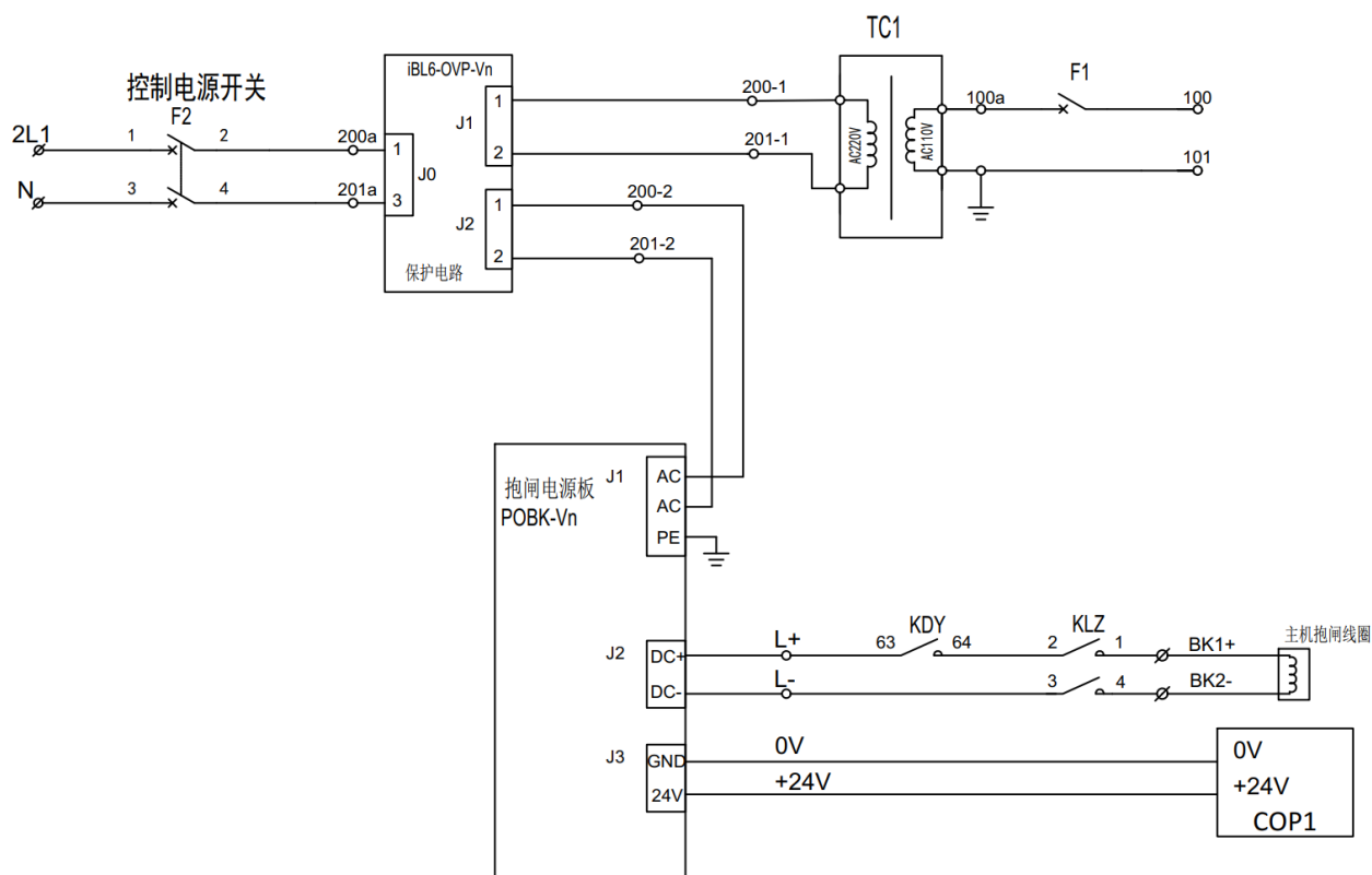
图 3.3 抱闸回路原理图
