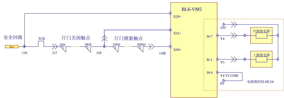
图 F7.3 新式外敞门+厅门电插锁
