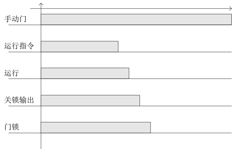
图 6.7 门锁断开时序图
