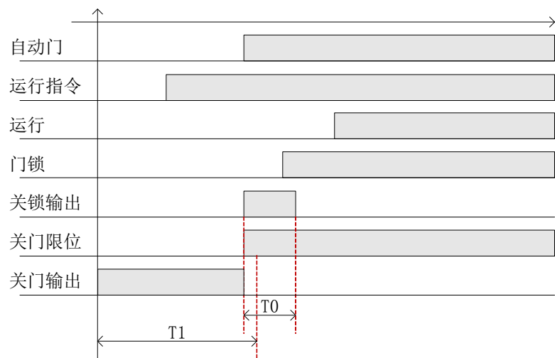
图 6.14 门锁吸合时序图
