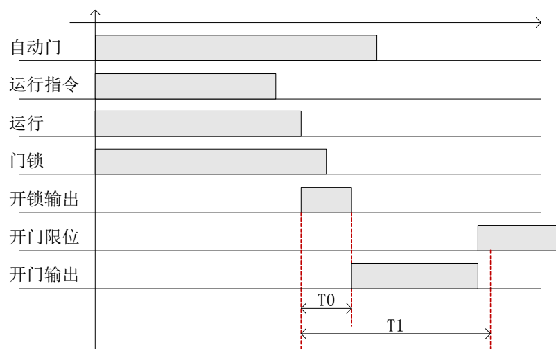
图 6.13 门锁断开时序图
