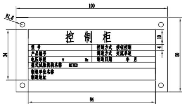
图 2.2 铭牌说明示意图
