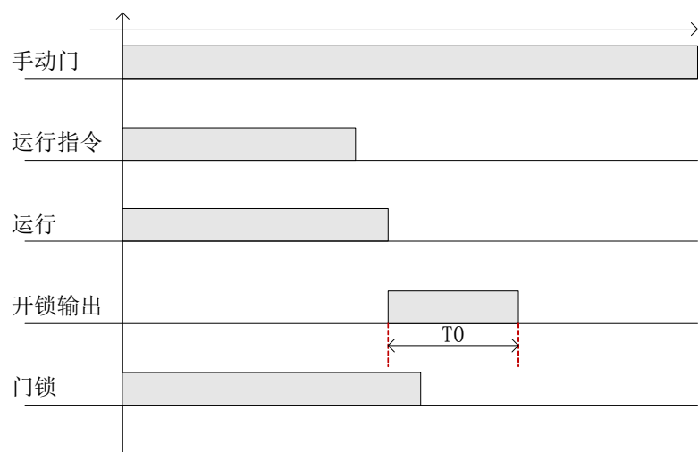
图 6.11 门锁断开时序图
