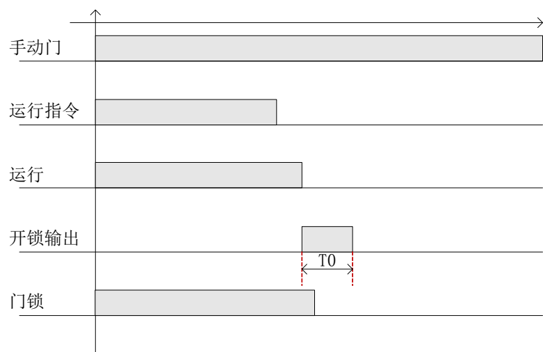
图 6.9 门锁断开时序图
