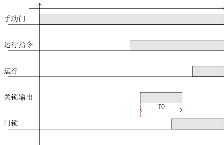
图 6.12 门锁吸合时序图
