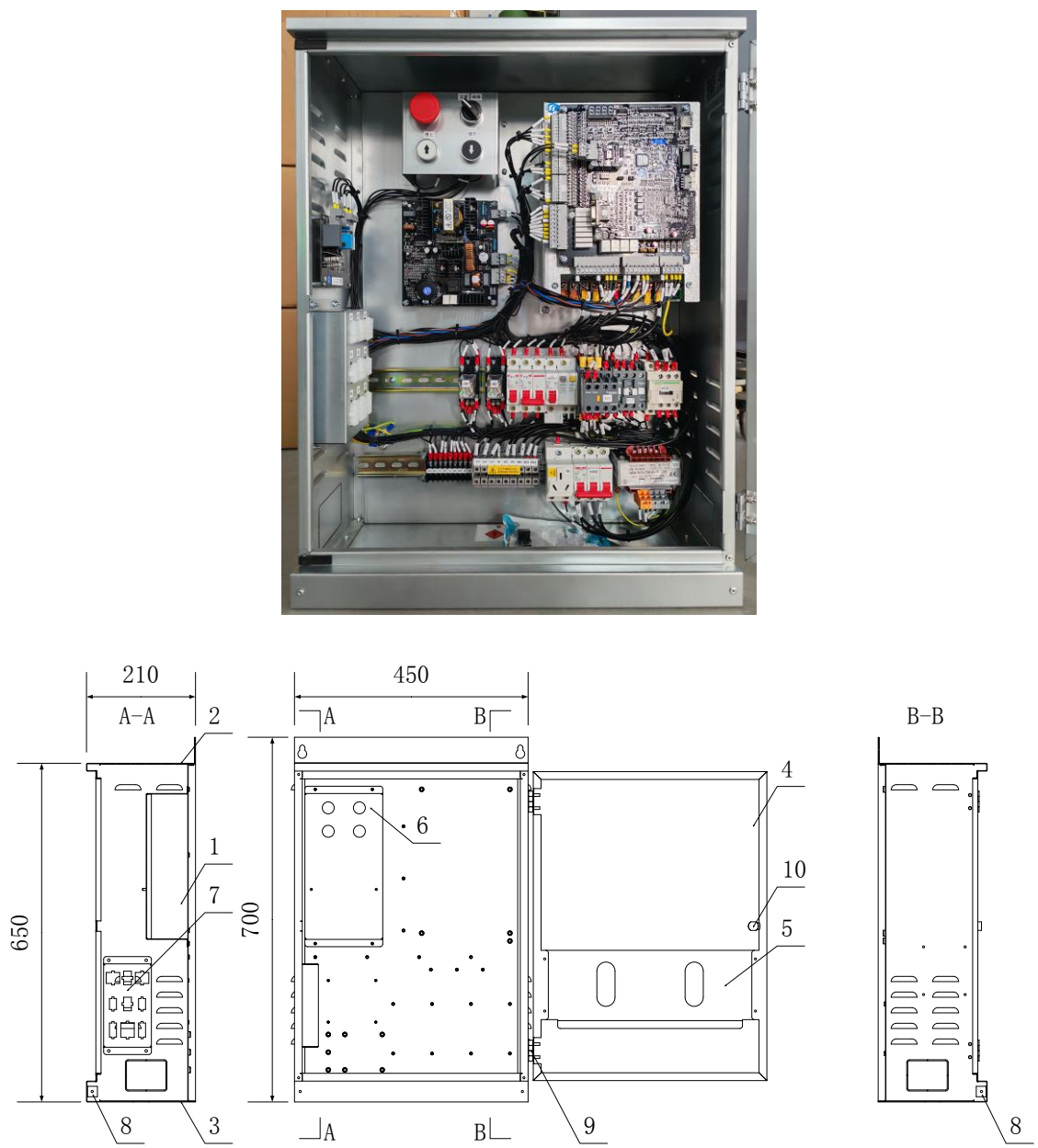
图 2.3 杂物梯控制柜外观及尺寸图（单位：mm）
