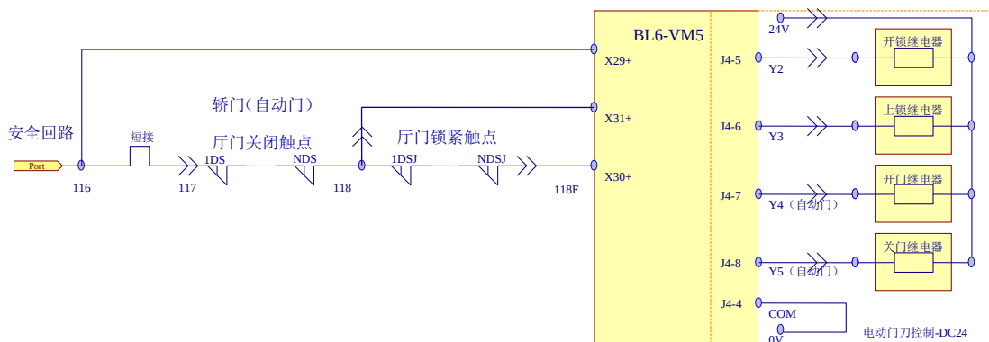
图 F7.2 上滑门+电动门刀方案
