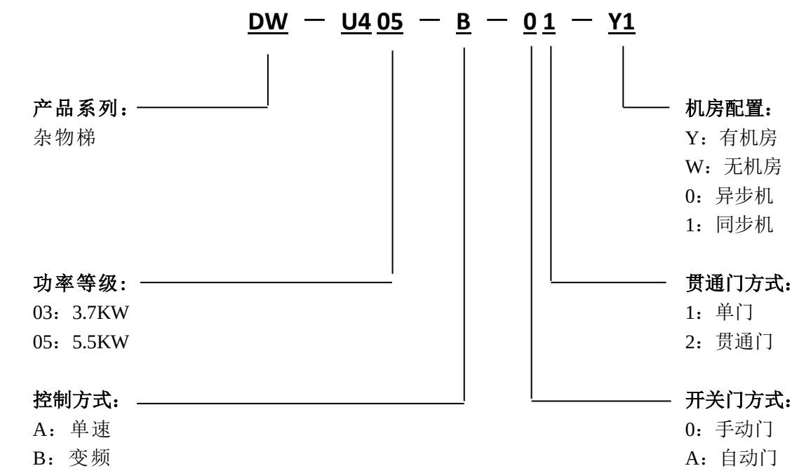
图 2.1 型号说明示意图
