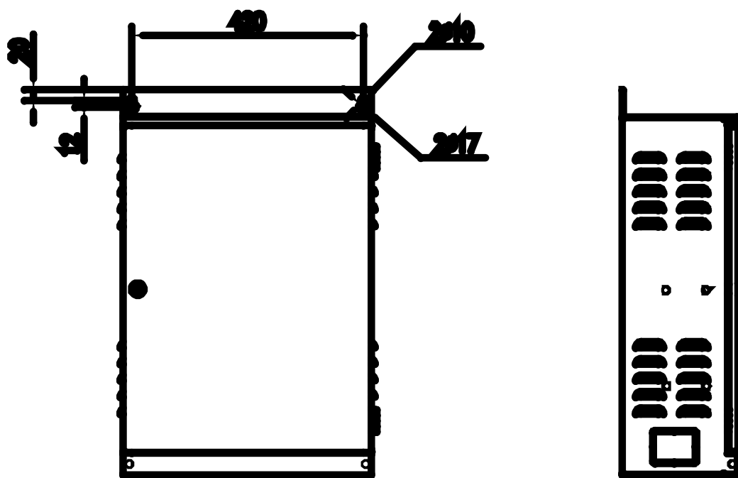
图 2.11 壁挂式安装示意图
