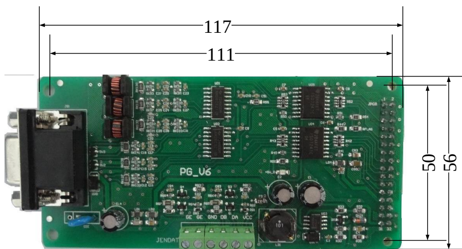
图 2.8 PG_V6 卡外型示意图
