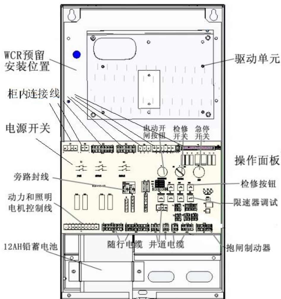
图 2.5 控制柜各部件名称与位置图
