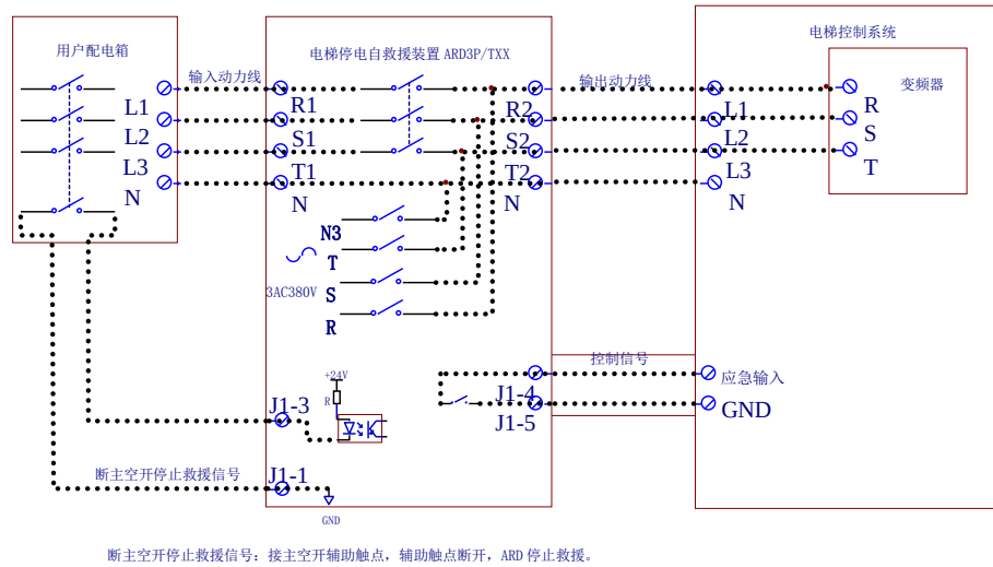
图 2.1 ARD3PXX 应用接线图
