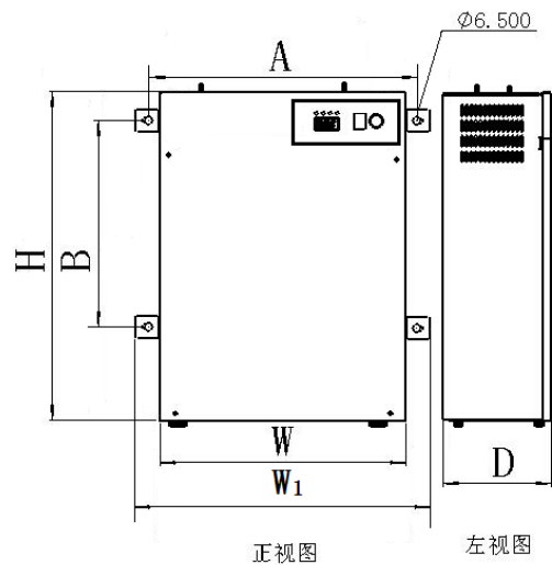
图 1.3 壁挂式尺寸图
