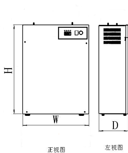
图 1.4 落地式尺寸图
