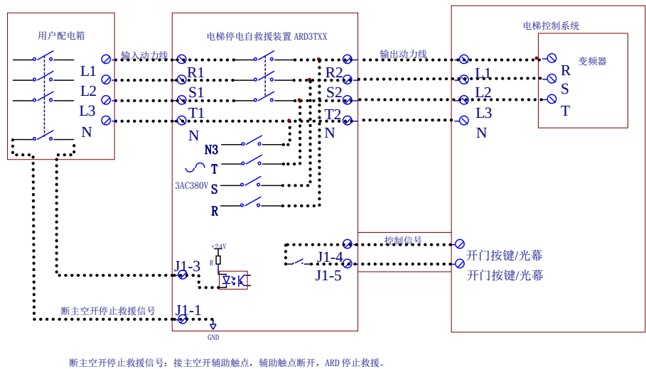
图 2.2 ARD3TXX 应用接线图
