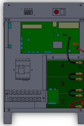
图 3.4 电池连线
