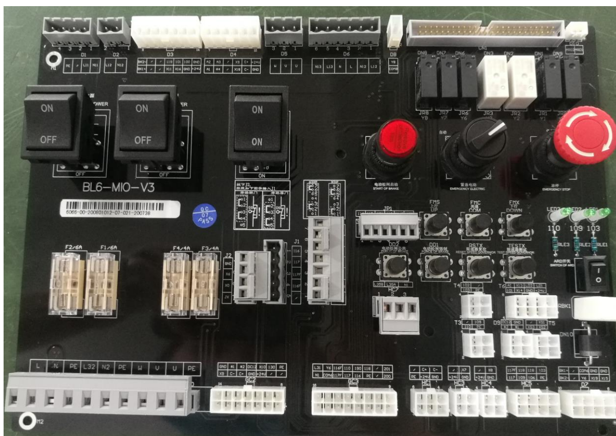
图 2.2 控制柜接口板
