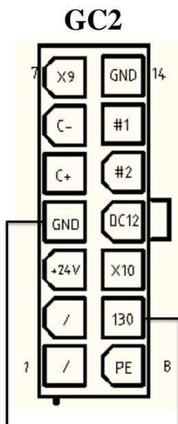
图 1.1 GC2-4 (GND) 与 GC2-9 (130) 短接
