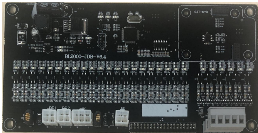
图 2.5 轿顶板
