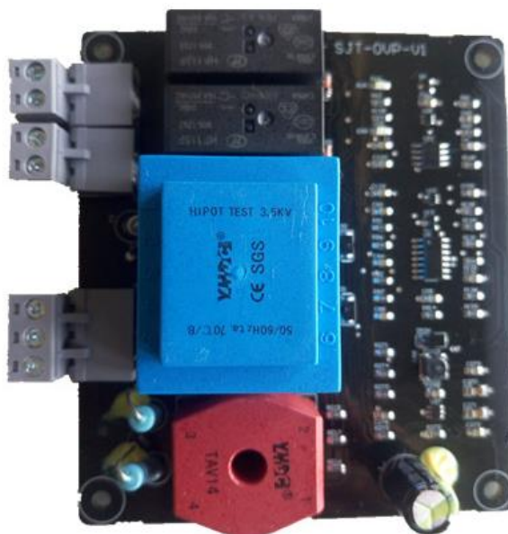
图 2.3 过压保护板
