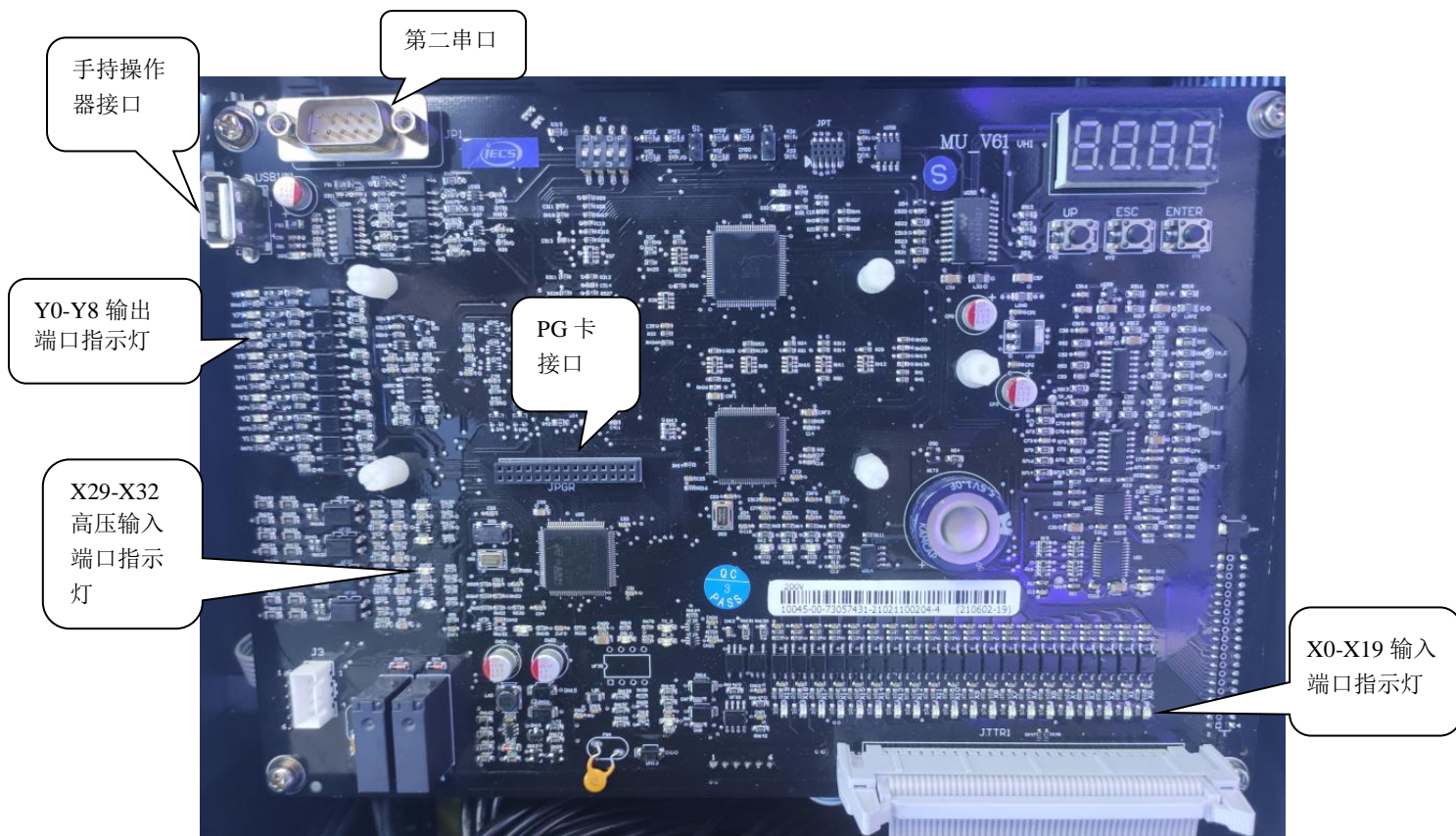
图 2.1 一体机主控板
