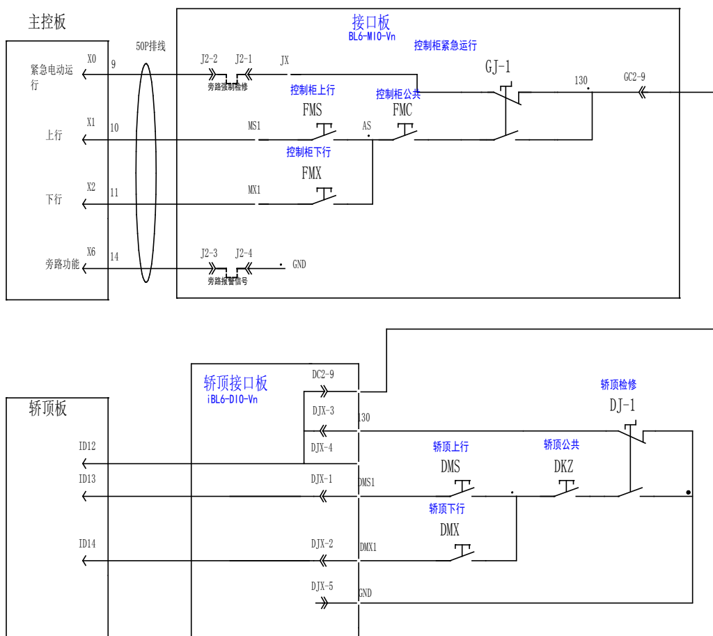
图 1.6 检修回路
